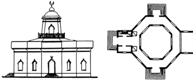
Рис. 2. «Образцовый» проект 1829 г. (из второго собрания ПСЗРИ)
