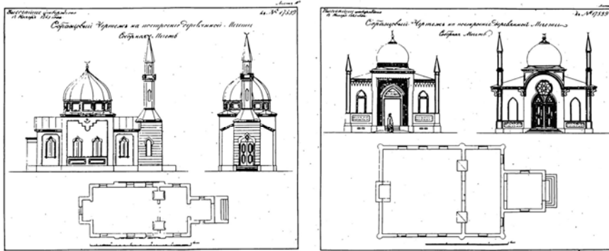
Рис. 3. Соборные мечети. «Образцовый» проект 1843 г. (из второго собрания ПСЗРИ)
