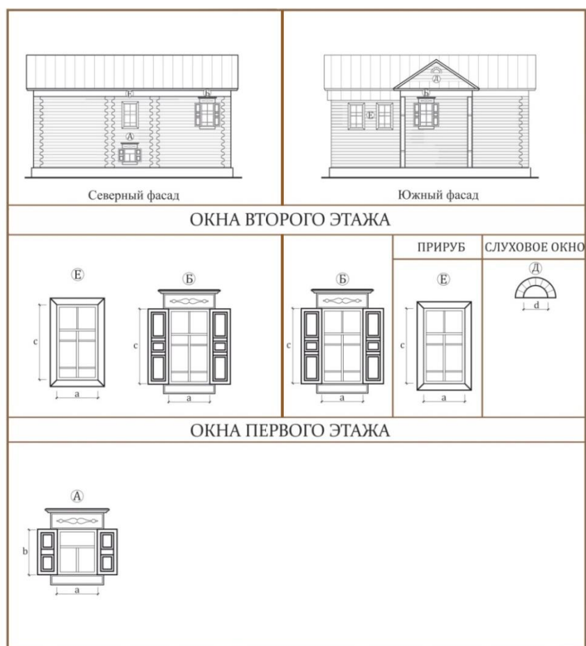
Рис. 2. Композиция фасадов жилого дома в стиле классицизм на ул. Белой, 10, в г. Томске. Выполнила Т.Ю. Козлова
