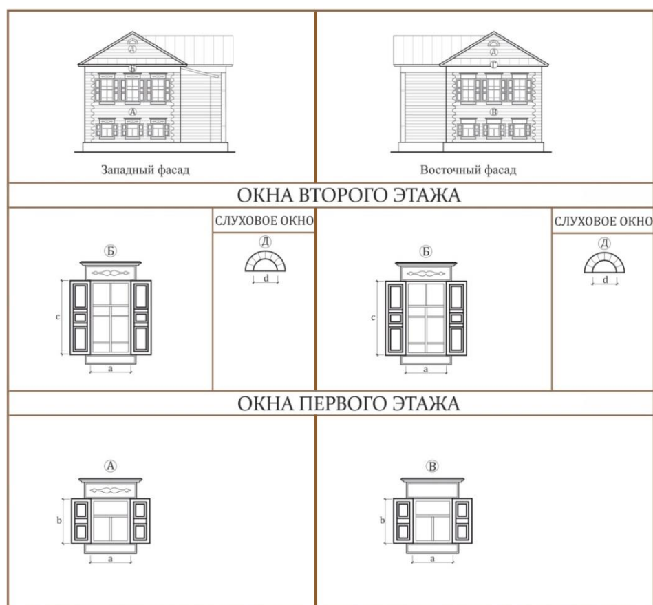
Рис. 1. Композиция фасадов жилого дома в стиле классицизм на ул. Белой, 10, в г. Томске. Выполнила Т.Ю. Козлова
