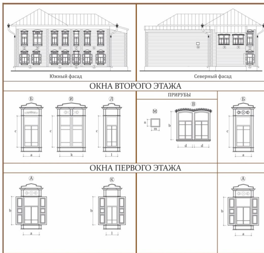
Рис. 4. Композиция фасадов жилого дома периода эклектики на ул. Р. Люксембург, 47, в г. Томске. Выполнила Т.Ю. Козлова
