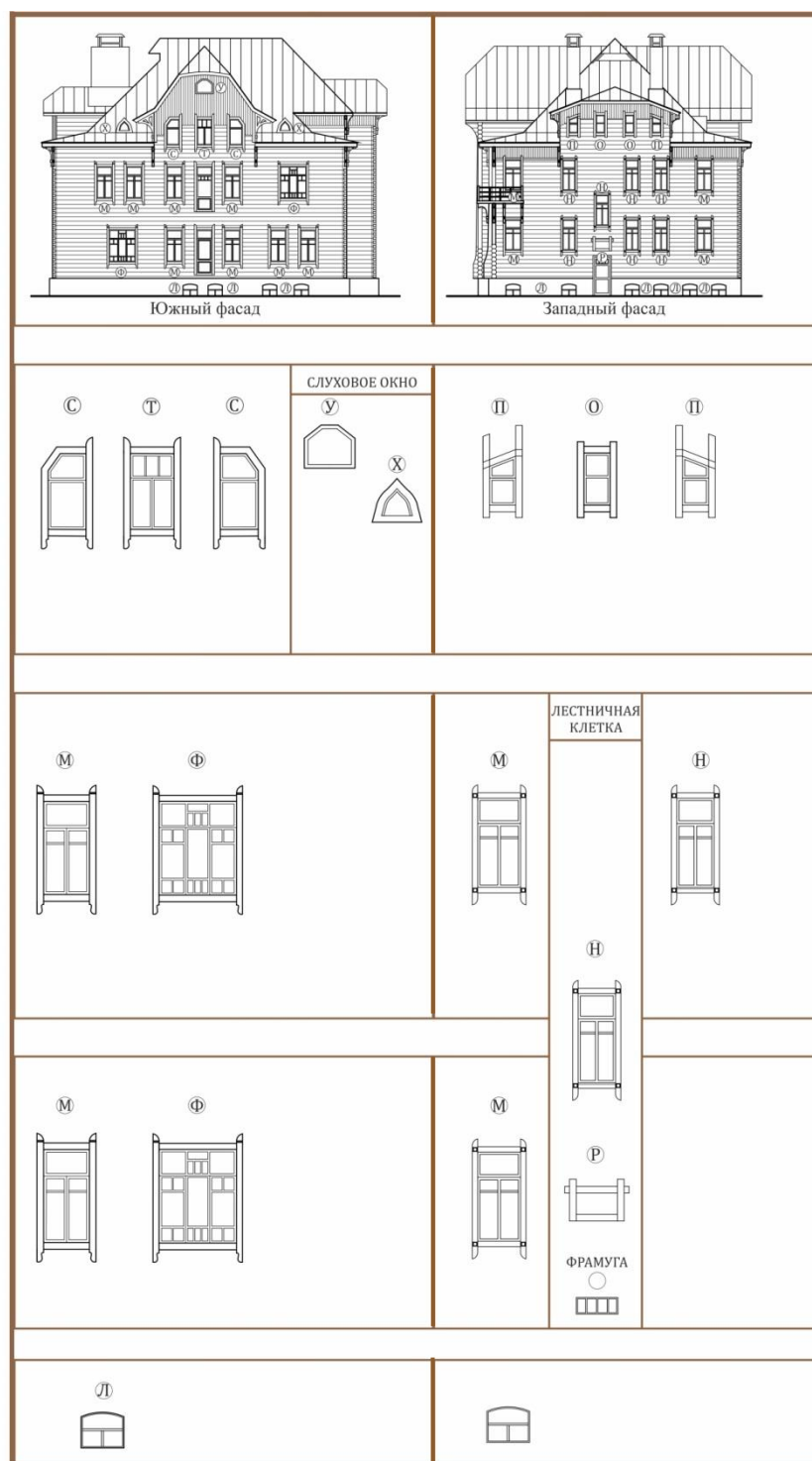
Рис. 6. Композиция фасадов особняка А.Д. Крячкова на пр. Кирова, 7, в г. Томске. Модерн. Выполнила Т.Ю. Козлова
