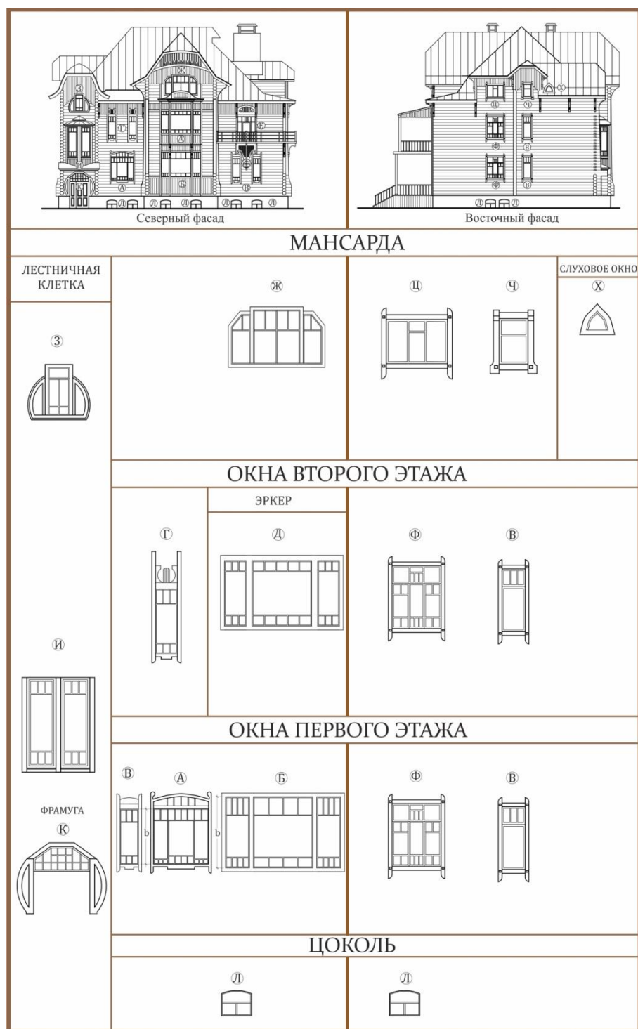
Рис. 5. Композиция фасадов особняка А.Д. Крячкова на пр. Кирова, 7, в г. Томске. Модерн. Выполнила Т.Ю. Козлова
