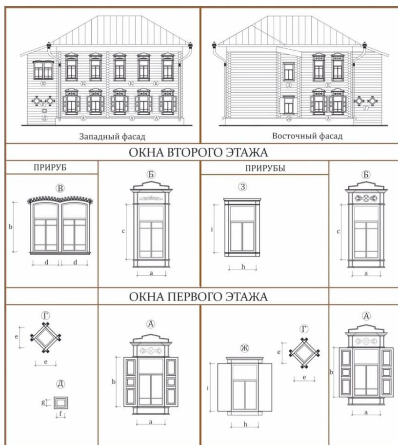
Рис. 3. Композиция фасадов жилого дома периода эклектики на ул. Р. Люксембург, 47, в г. Томске. Выполнила Т.Ю. Козлова
