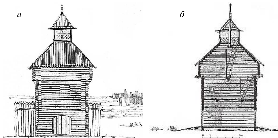
Рис. 1. Нарымский острог в конце XVII в. Графическая реконструкция Н.В. Шагова: а – Воротная южная башня. Вид со стороны острога; б – разрез
