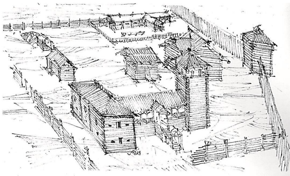
Рис. 3. Усадьба воеводы И.Л. Скобелцина 1643 г. и служилых людей в Нарымском остроге. Графическая реконструкция Н.В. Шагова, 2009 г.
