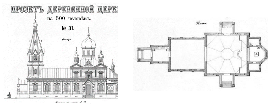
Рис. 1. Типовой проект деревянной церкви № 31 из Атласа планов и фасадов церквей 1889 г. [5] Fig. 1. Standard design for wooden church No. 31 from the Atlas of Church Plans and Facades, 1889
