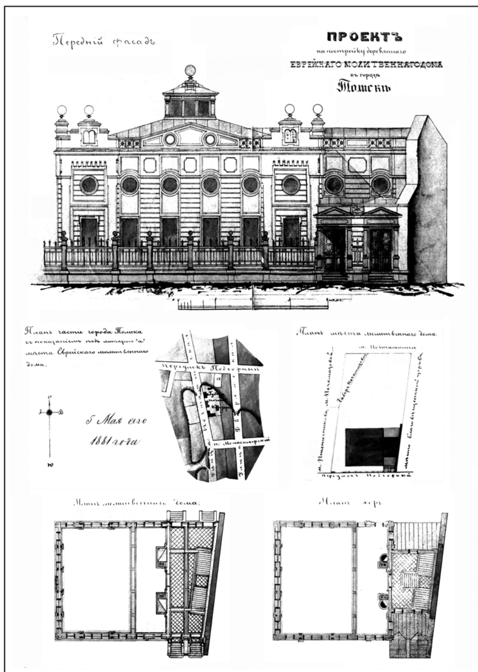
Рис. 2. Каминерская синагога в Томске (1881–1883). Проект синагоги, подписанный и.о. губернского архитектора А.П. Бетхером (май 1881 г.): главный фасад с пер. Подгорного; ситуационный план, план участка; планы 1-го и 2-го этажей (из фондов Государственного архива Томской области)
