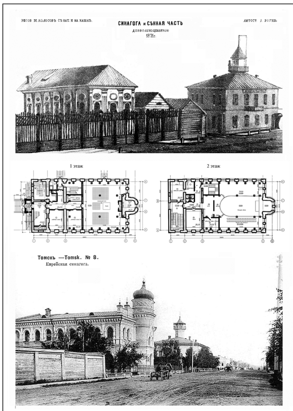
Рис. 1. Синагога на ул. Магистратской в Томске. Литография художника М. Колосова, 1871 г. (из фондов ТОКМ); планы 1-го и 2-го этажей (чертежи выполнены в ОАО «СИ «Сибспецпроектреставрация», арх. Е.Ю. Хатажукова, 2008 г.); почтовая открытка «Еврейская синагога» (из коллекции А.Б. Казачкова)
