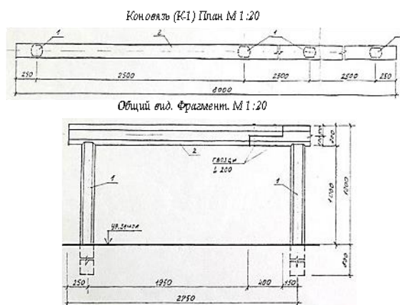
Рис. 10. Чертеж коновязи. Спецпроектреставрация, г. Томск, 1987 г.
