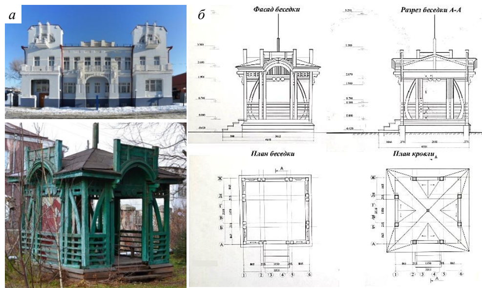
Рис. 8. Беседка в стиле модерн по ул. III Интернациональной, г. Бийск (а); чертежи беседки из дипломной работы А.П. Семина (б), материалы архива кафедры РИРАН ТГАСУ, 2006 г.
