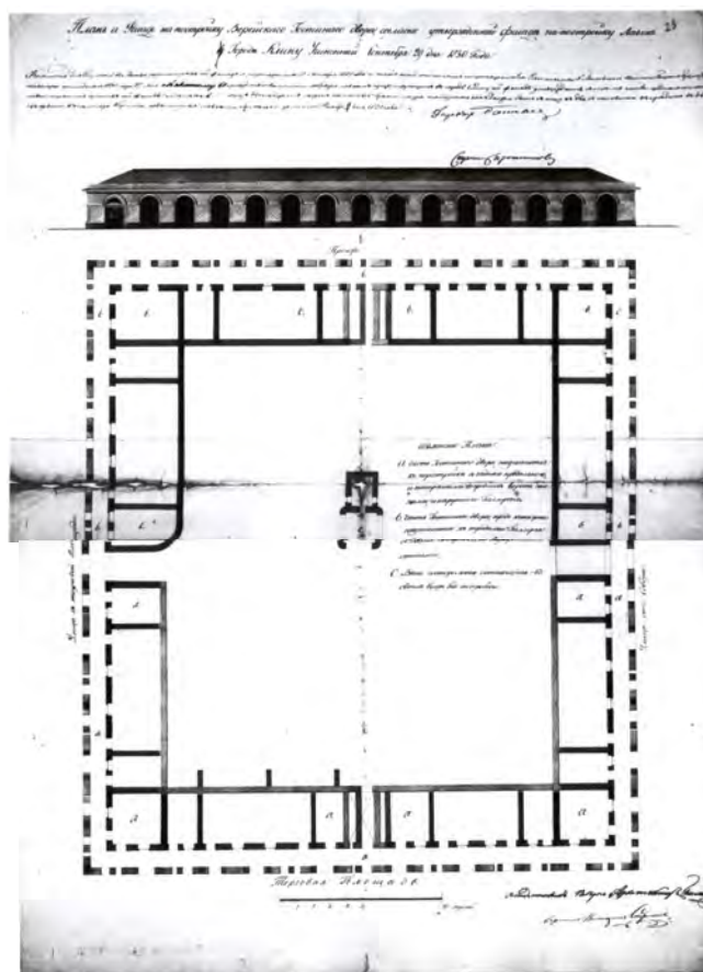
Рис. 1. Проект перестройки гостиного двора в Верее 1831 г. ЦИАМ
