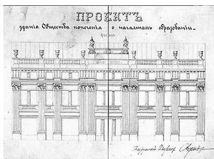
Рис. 9. Проект дома Общества попечения о начальном образовании. Автор архитектор С.Г. Дриженко. 1913 г. [14]
