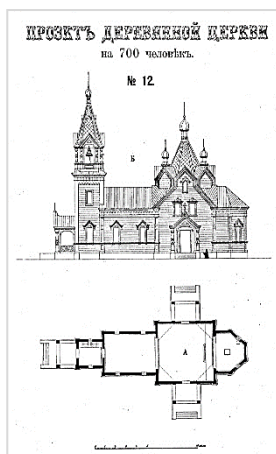
Рис. 25. Проект деревянной церкви на 700 чел. № 12 [7, с. 17]
